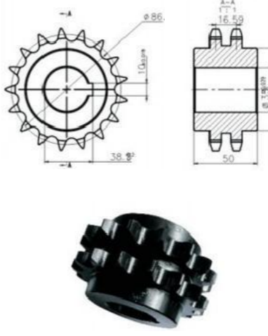
驱动电机链轮轴上用
