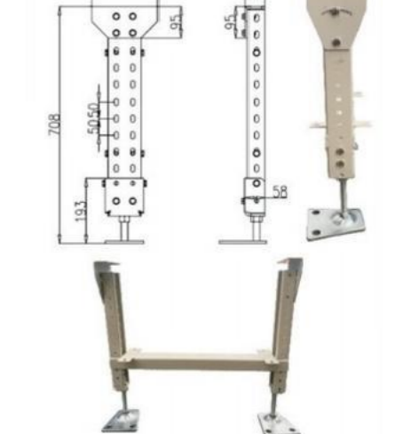
⑮支腿
