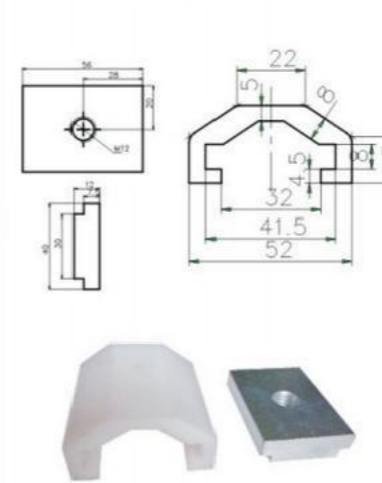
⑤滑块套件
