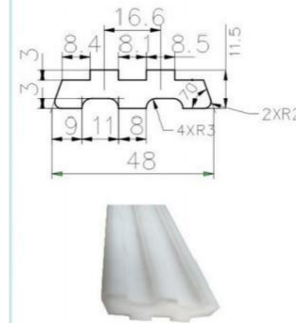
④托条
