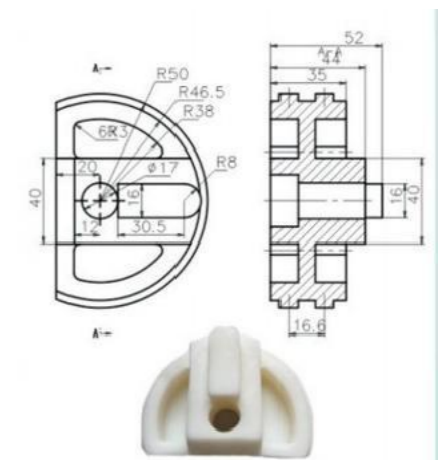
③涨紧轮
